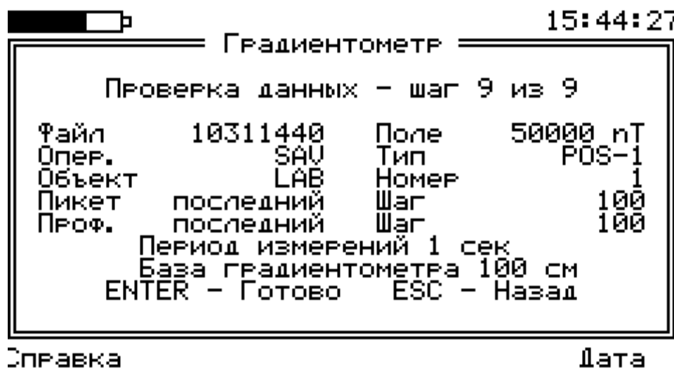
Рис. 34. Проверка параметров при открытии файла в режиме градиентометра
