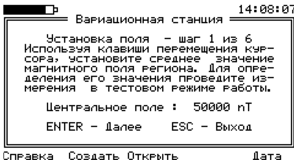
Рис. 15. Установка поля в режиме вариационной станции
