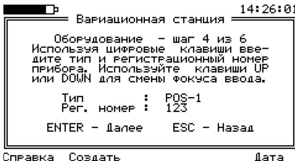
Рис. 18. Ввод типа и регистрационного номера используемого магнитометра
