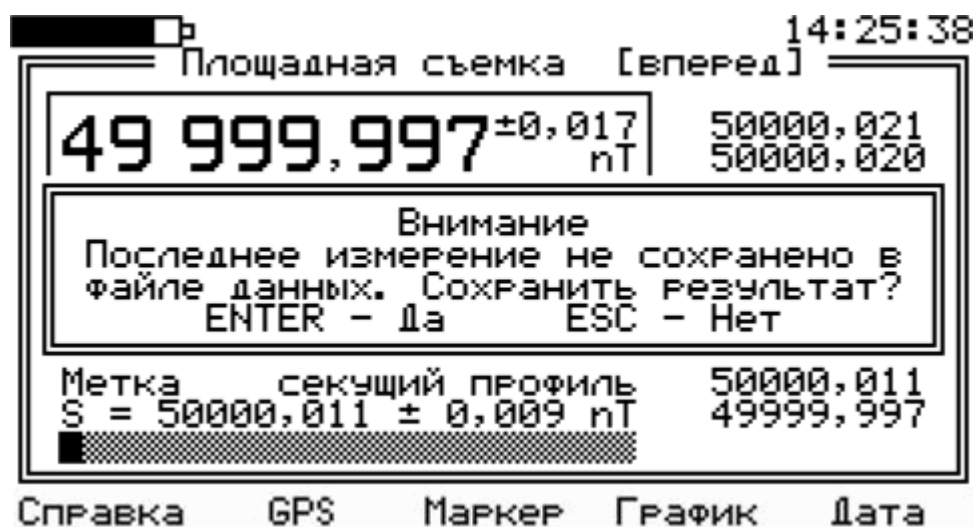
Рис. 31. Запрос на сохранение результата измерения
