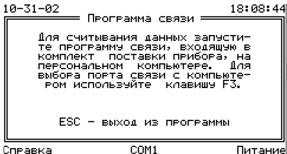
Рис. 42. Диалоговое окно программы связи с компьютером
