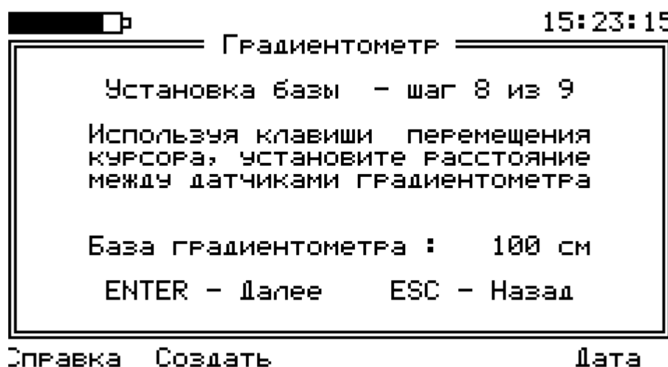
Рис. 32. Определение базы градиентометра
