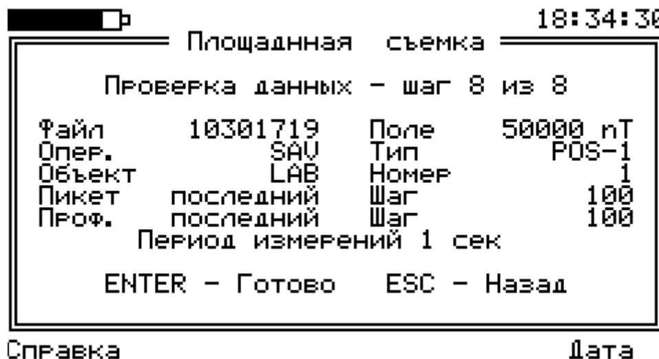
Рис. 27. Проверка открытия файла в режиме площадной съемки
