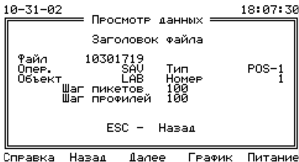
Рис. 41. Просмотр параметров съемки, сохраненных в файле данных
