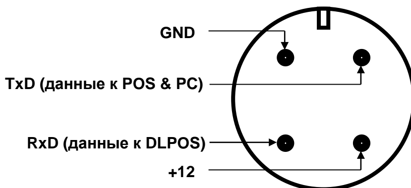
Рис. 3. Распайка разъемов внешних устройств накопителя данных DLPOS
