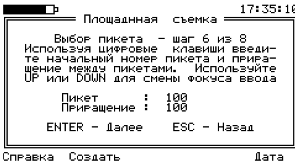
Рис. 24. Привязка к пикетам в режиме площадной съемки
