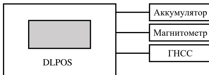
Рис. 5. Схема подключения магнитометра и ГНСС-приемника к DLPOS
