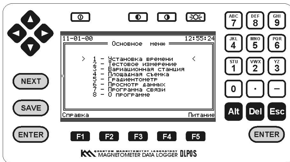
Рис. 4. Внешний вид лицевой панели накопителя данных DLPOS
