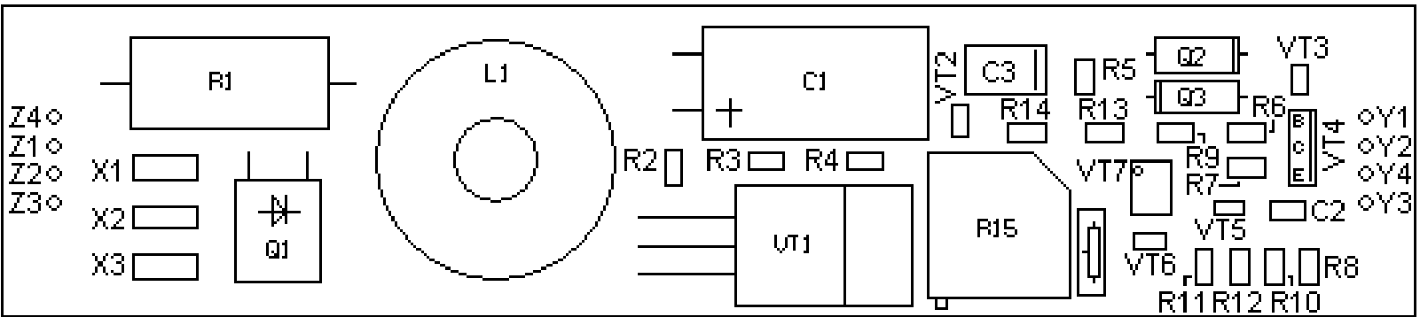
Блок питания
