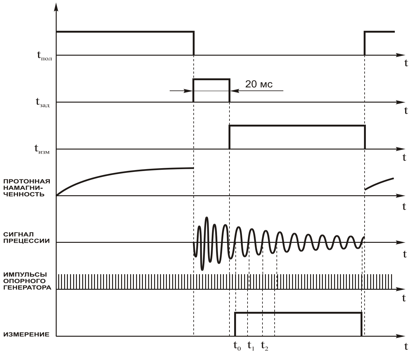
Рис. 2. Временная диаграмма работы LOM-2
