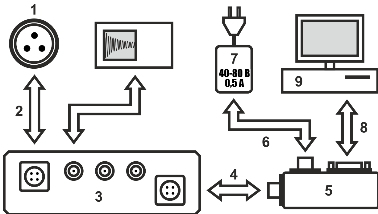
Рис. 1. Сборка магнитометра LOM-2
