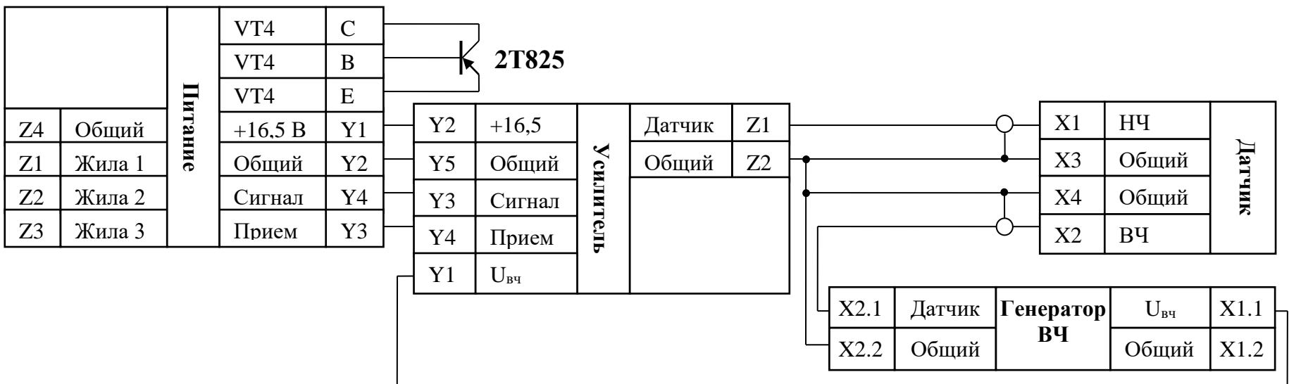
Блок схема скважинного зонда
