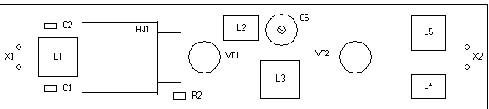
ВЧ-генератор
